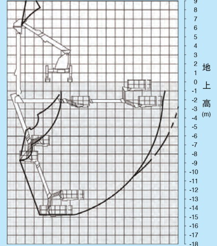
アウトリガ中間1張出
