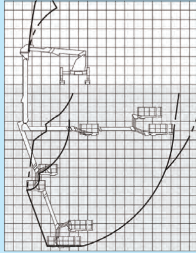
アウトリガ中間2張出
